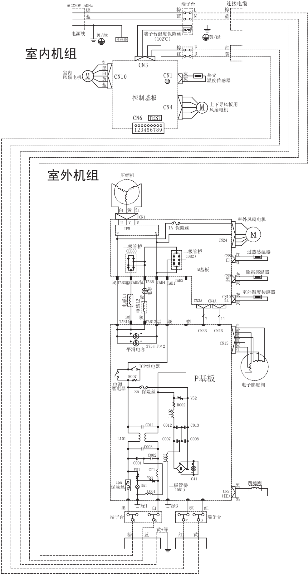
原理图 室内外电气原理图
