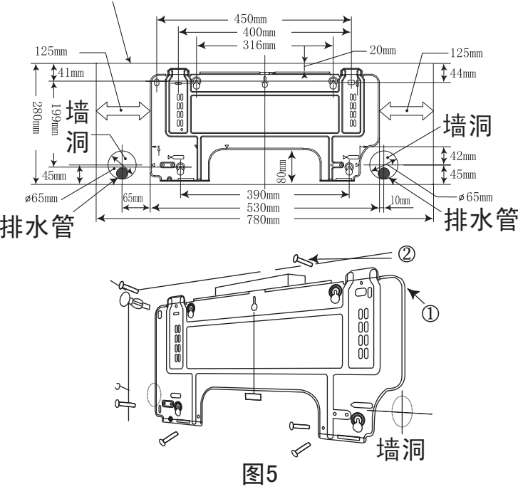
室内机外形线
