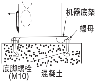
图4 安装基础
