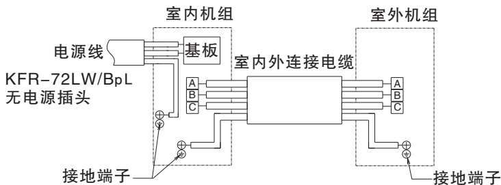
图15 室内外电气连接图
