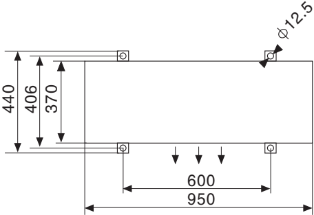
图3底脚螺栓位置
