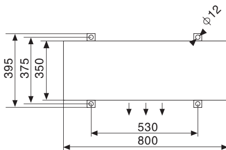
图5 底脚螺栓位置
