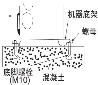
图4 安装基础
