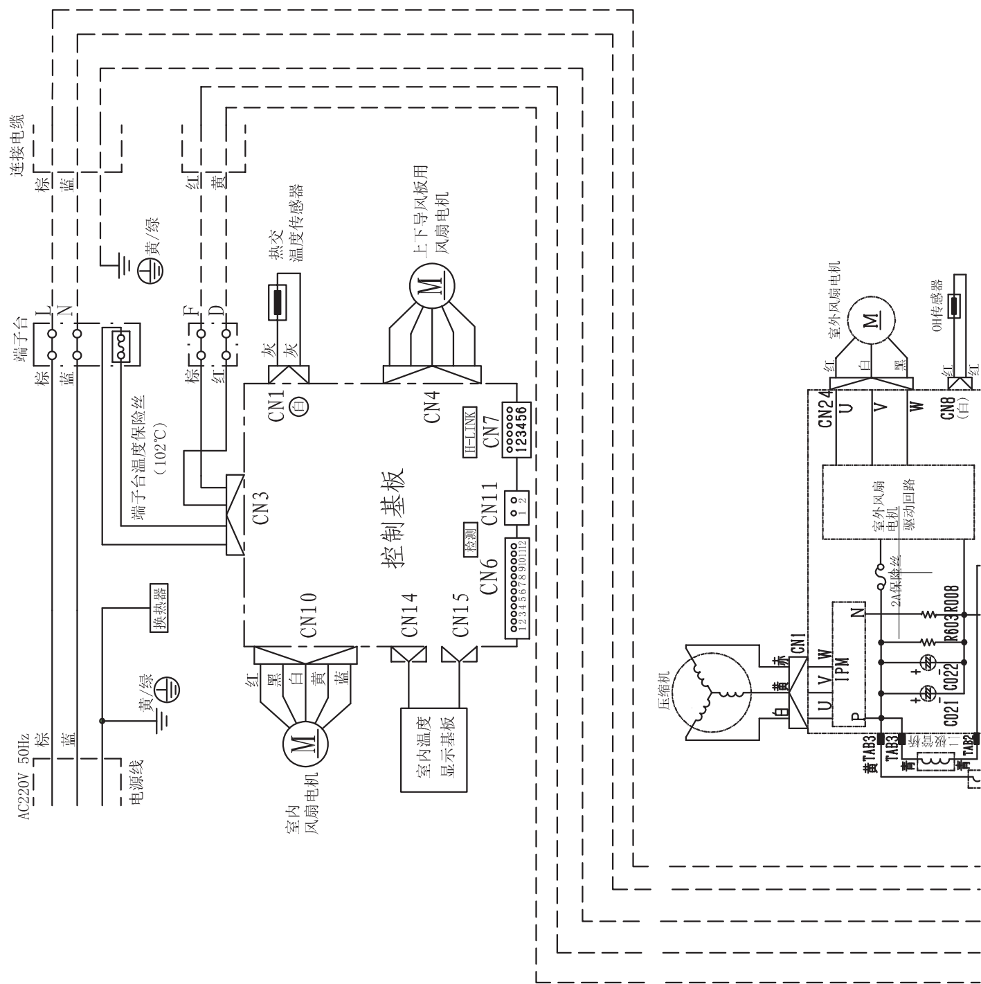
室内外电气原理图 (RAS/C-25DVY、RAS/C-35DVY、RAS-35DVYB/RAC-35DVY)
