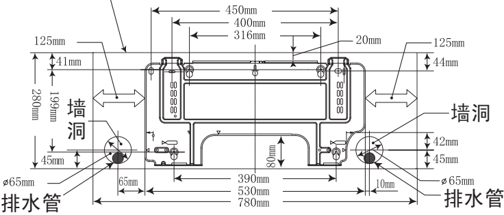
室内机外形线
