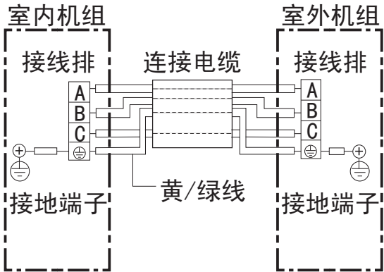
图27 室内外电气连接图
