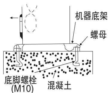
图4 安装基础
