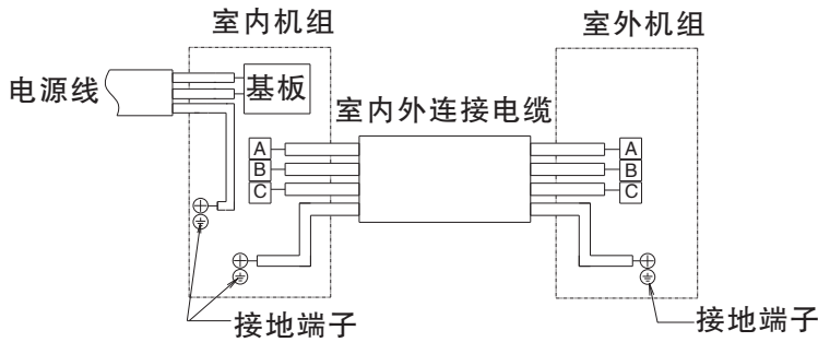
图15 室内外电气连接图
