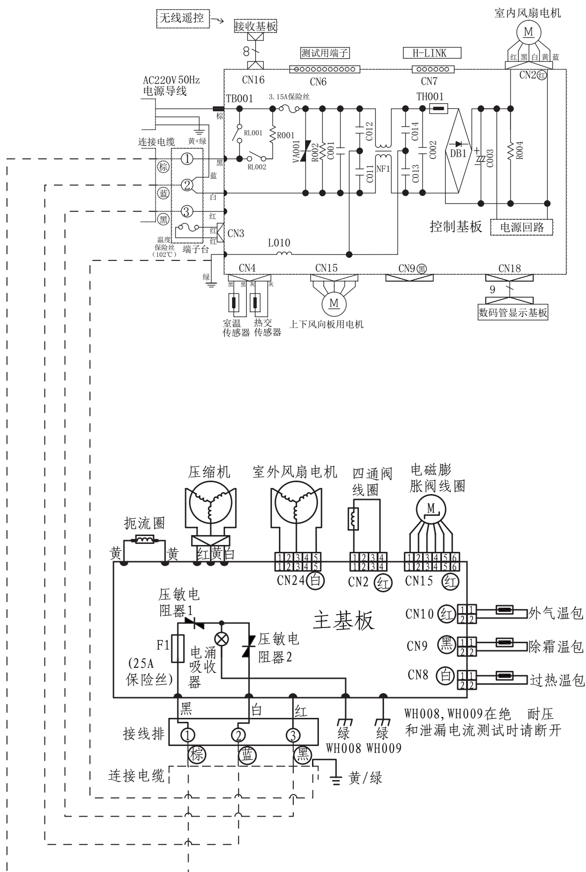
室内外电气原理图
