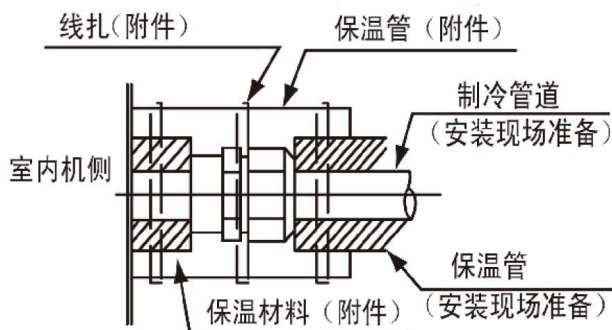
图20 管的保温
