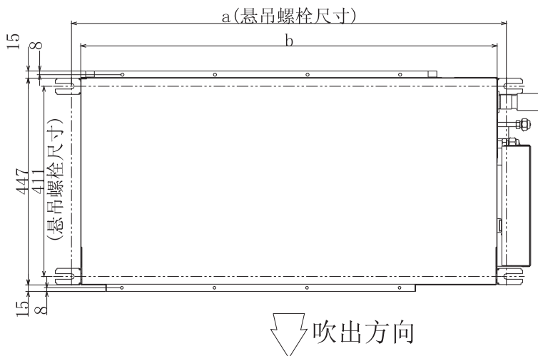
图3 悬吊螺栓 (单位: mm)
