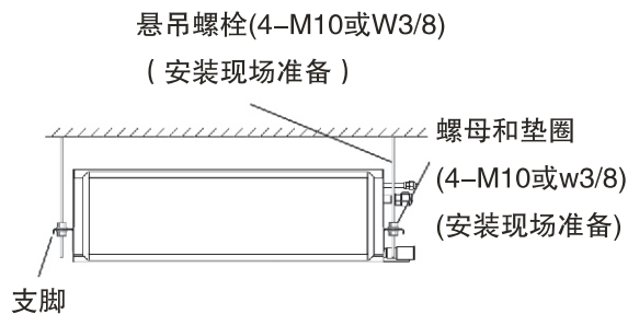
图4 室内机安装
