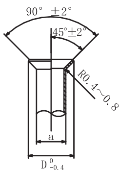
图18 扩口加工
