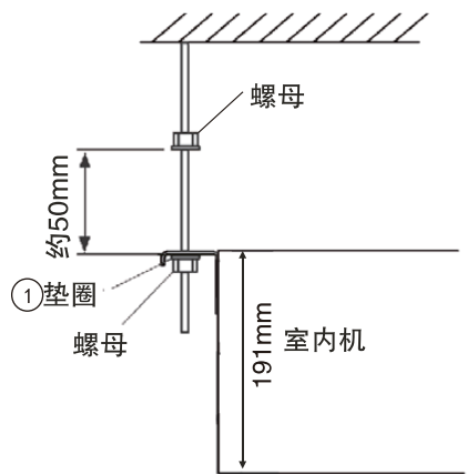
图5 悬吊螺栓和螺母
