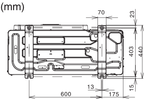
图13-1 底脚螺栓位置
